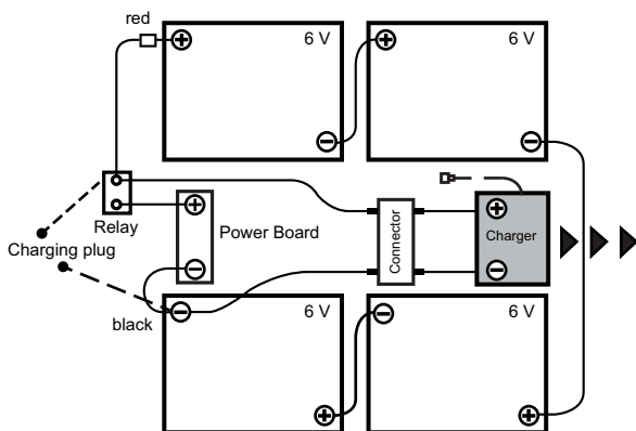
Схема на свързване на батерията
